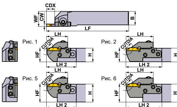
Показана правая державка.
