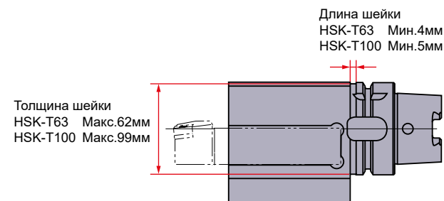
Стандарт токарного инструмента HSK-T (пример)
